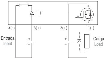
Diagrama Elétrico / Schematic
